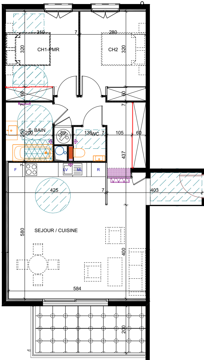
PLAN APPARTEMENT
